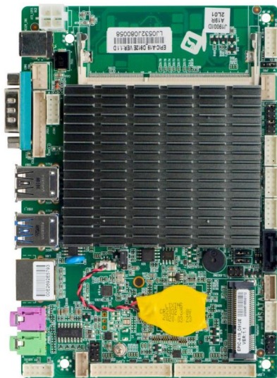
EPIC-A19_D912E VER:1.1 主板正面图
