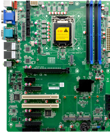
Z270DM VER:1.0 正面图
