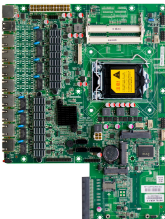
H87SL VER:1.3 主板正面图
