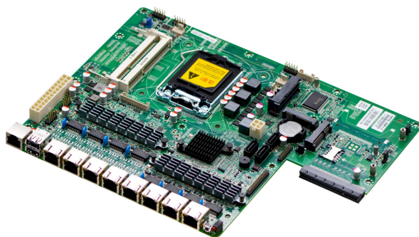
H87SL VER:1.3 主板侧面图
