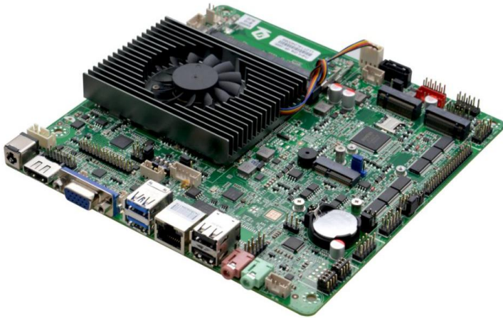
ITX-B110_C316L VER:1.0 侧面图
