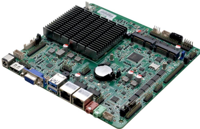
ITX-B413_J1210L VER:1.0 主板侧面图
