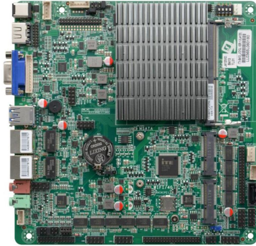
ITX-B413_J1210L VER:1.0 主板正面图
