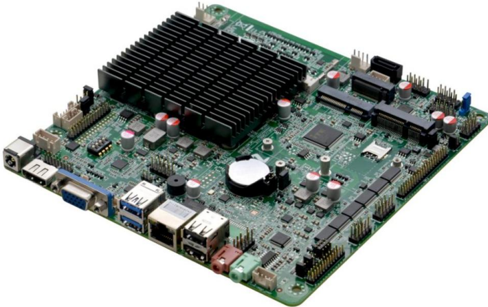
ITX-B346_J116L VER:1.2E 主板侧面图
