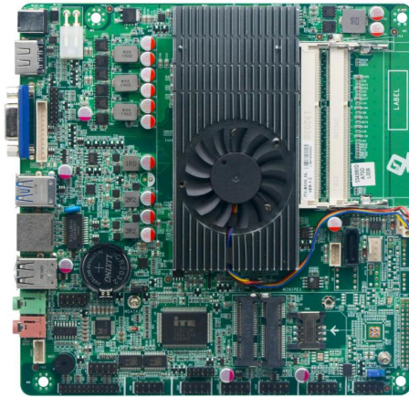
ITX-B530_NL VER:1.0 主板正面图
