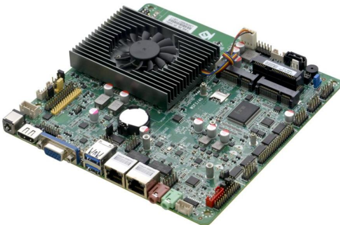
ITX-B430_I526L VER:1.6 主板侧面图
